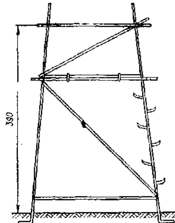
Рис. 27. Металлическая переносная площадка для наблюдения с пирамид-штативов. Изготавливается из уголкового стали (50×50×5 и 35×35×4)
