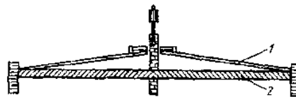
Рис. 29. Тур со съемной визирной целью 1 - крыша; 2 - перекрытие (балка)
