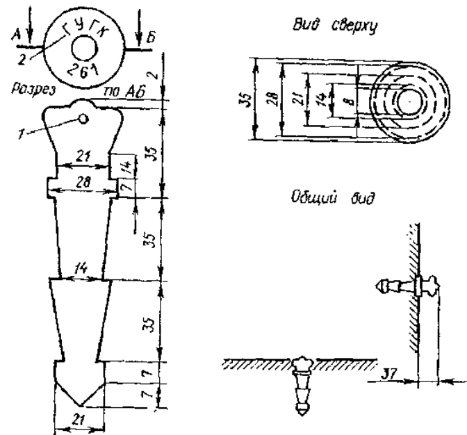
Рис. 37. Стенной знак пункта полигометрии 2, 3, 4 классов, 1 и 2 разрядов. Тип 8 г. р.
