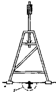
Рис. 30. Пирамида-штатив со съемной визирной целью 1 - марка триангуляционная
