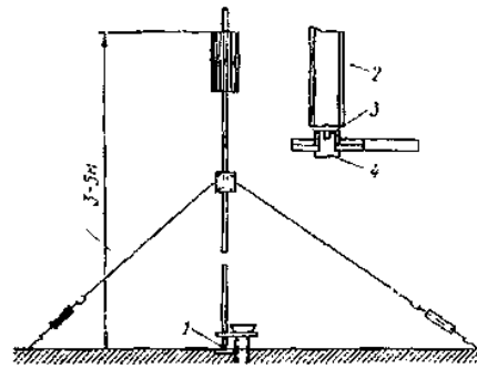
Рис. 31. Съемная металлическая веха с визирным цилиндром 1 - центр пункта; 2 - веха; 3 - отверстие (центр пункта); 4 - болт
