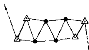
Рис. 21 Центральная система
