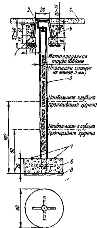
Рис 33. Центр пункта триангуляции, полигонометрии, трилатерации 2, 3, 4 классов для районов глубокого промерзания грунта (свыше 1,5 м) и для районов многолетней мерзлоты. Тип 2 г. р.
