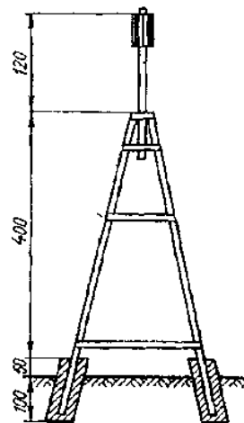
Рис. 25 Четырехгранная пирамида (из уголковой стали)
