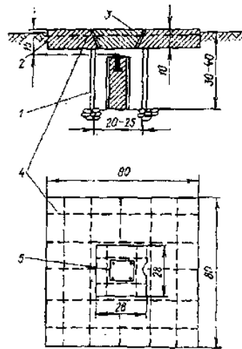
Рис. 38. Наружное оформление мест расположения пункты триангуляции, полигометрии, триангуляции 2, 3, 4 класса на незастроенной территории.
