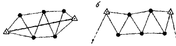
Рис. 24 Цепочки треугольников между двумя пунктами
