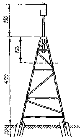
Рис. 26. Пирамида-штатив из уголковой стали (50×50×5 или 35×35×4) со съемной малофазной визирной целью с высотой до инструментального столика от 1,2 до 0,4 м.
