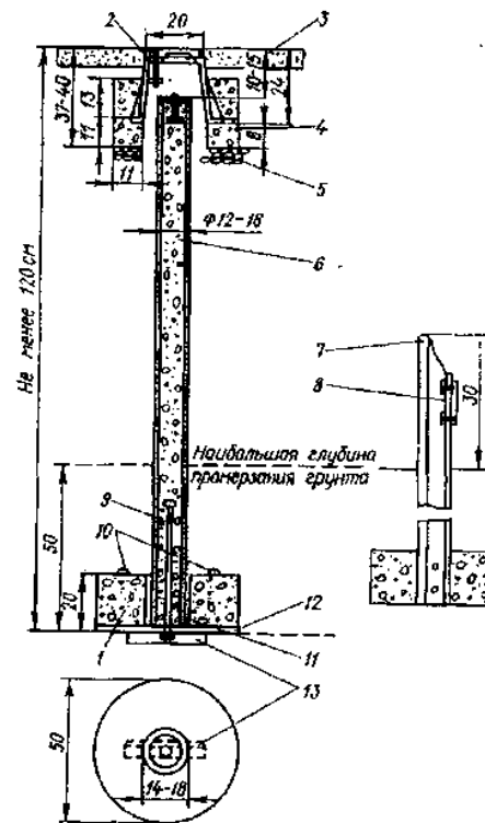
Рис. 32. Центр пункта триангуляции, полигонометрии, трилатерации 2, 3, 4 классов для районов неглубокого (до 1,5 м) промерзания грунта. Тип 1 г. р.
